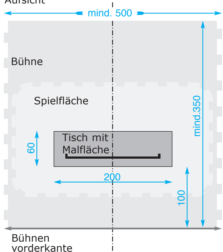
Aufsicht
